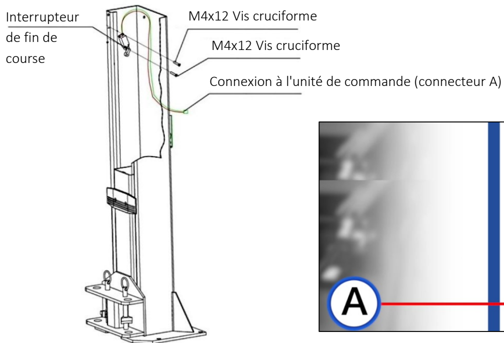
Figure : Montage de l'interrupteur de fin de course
