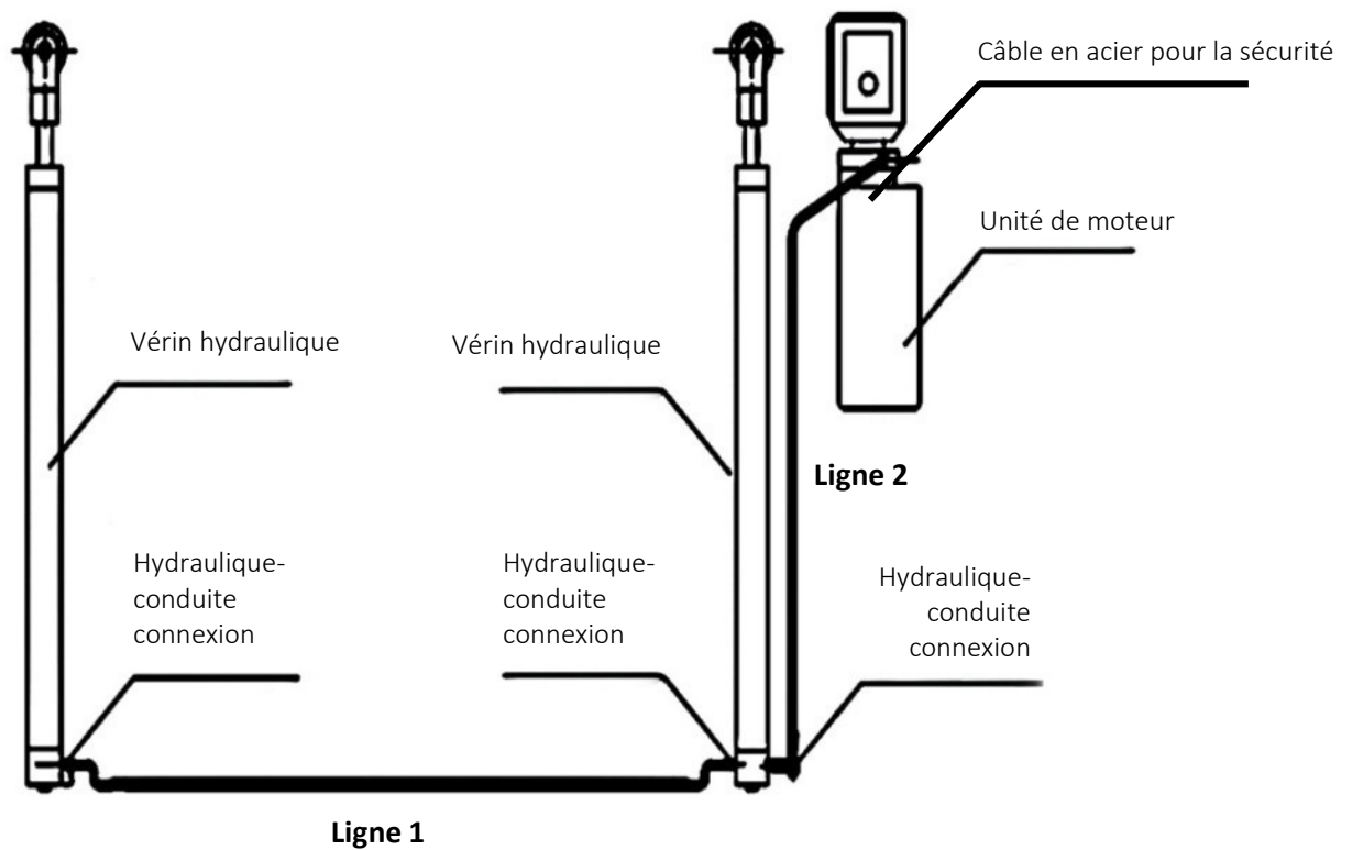
Figure : Montage de la conduite hydraulique
