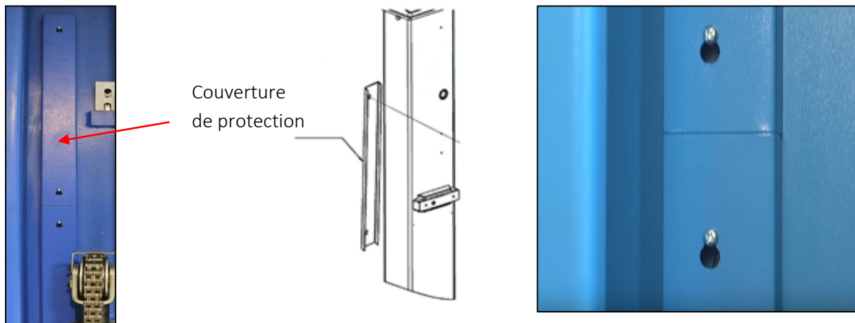
Figure : Mise en place des couvercles de protection des interrupteurs de fin de course
