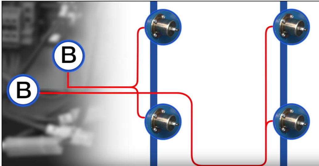
Figure : Connexions du déverrouillage de l'électroaimant
